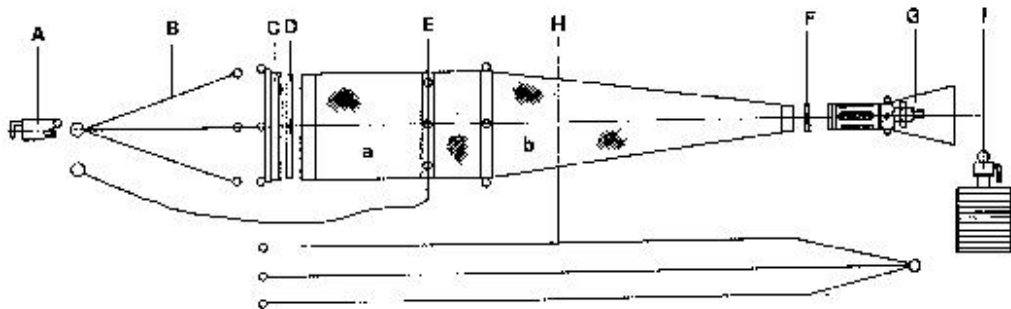
WP-2浮游生物分层网结构示意图
